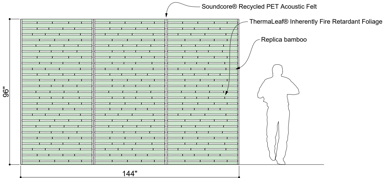
② ELEVATION 2
